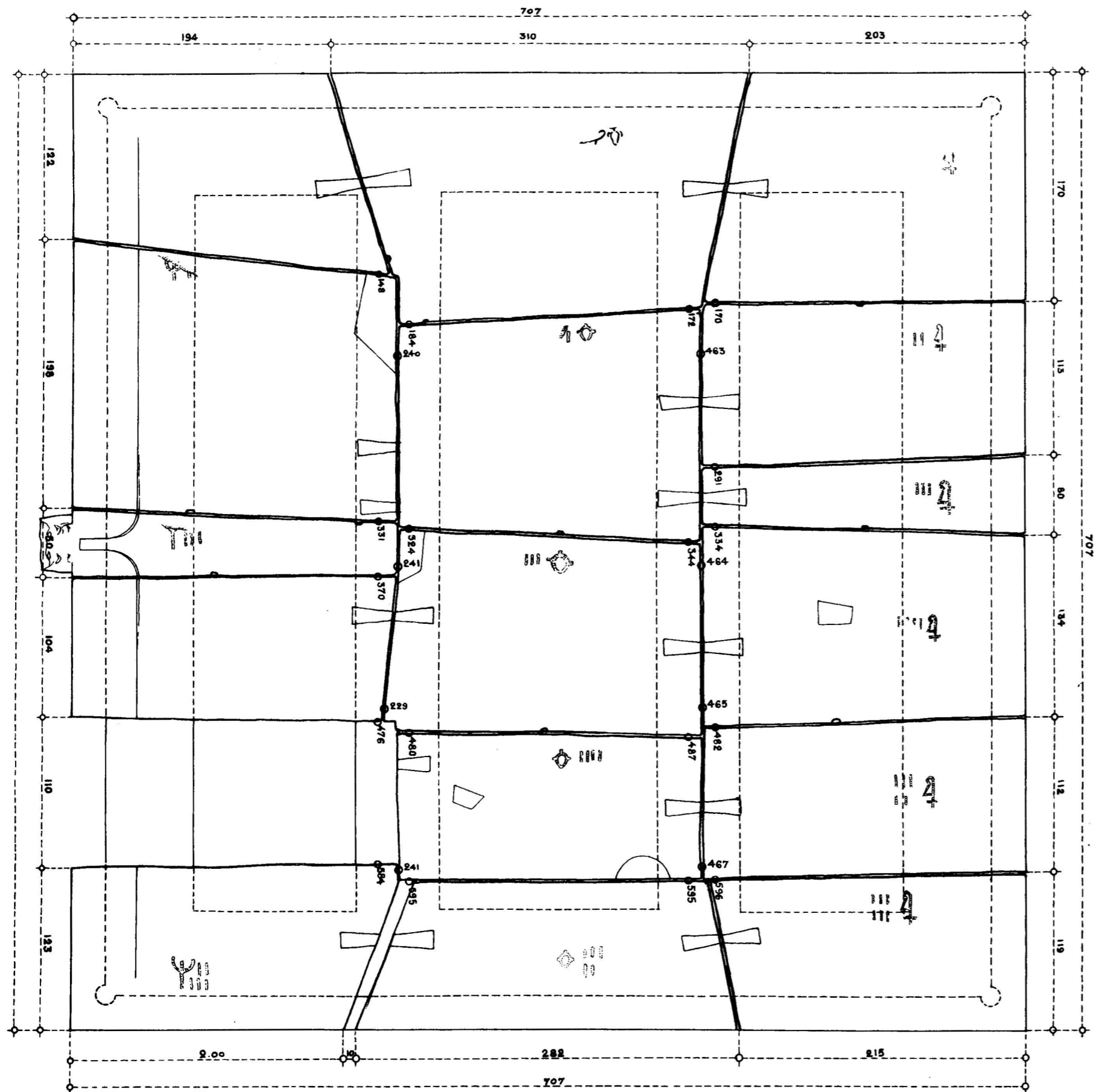
PLAN DES ARCHITRAVES
