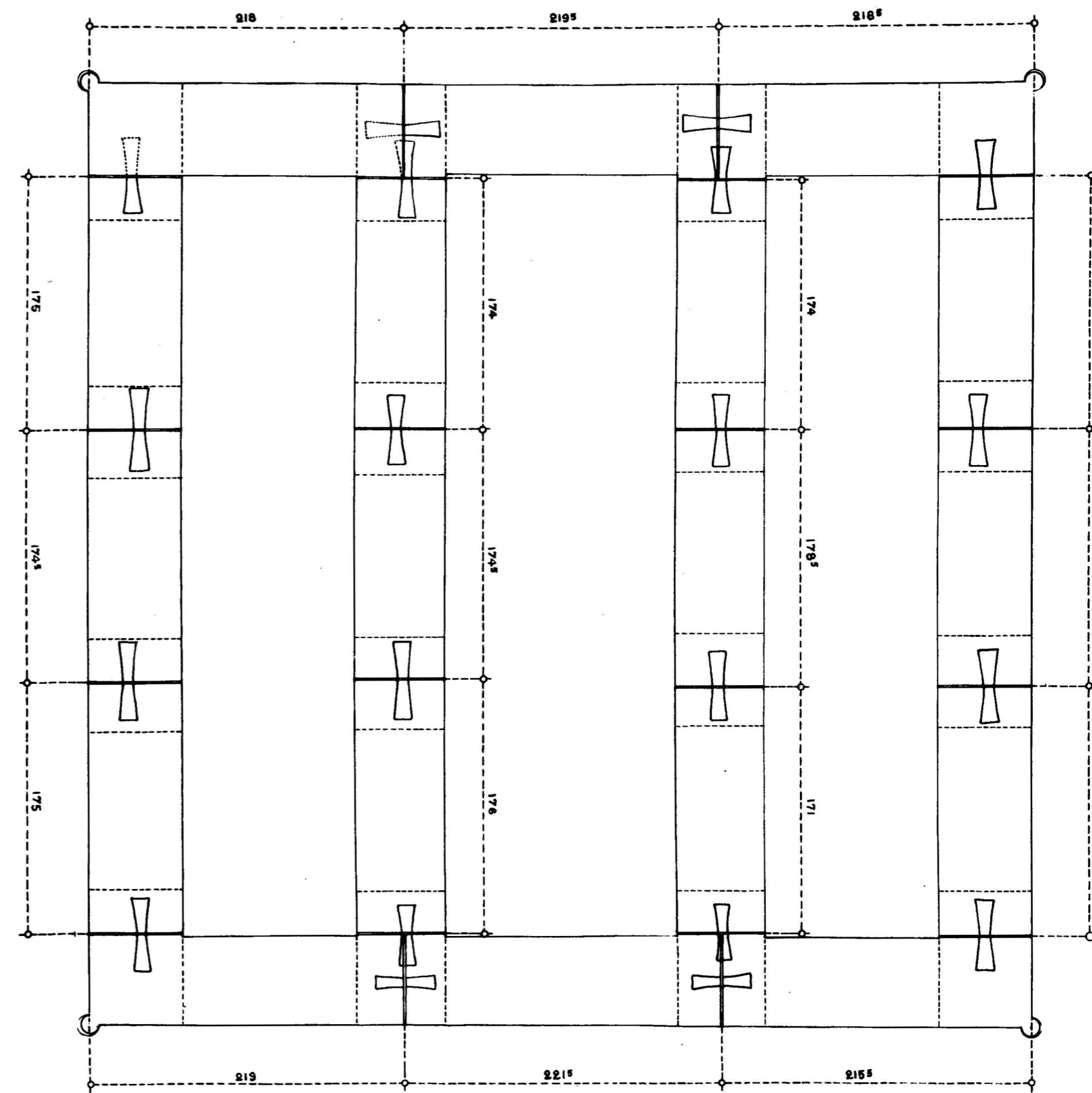
PLAN DES DALLES DE COUVERTURE
